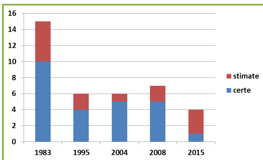
Figura 9. Evoluzione della popolazione di Lanario nel Lazio nel periodo 1983-2015.
