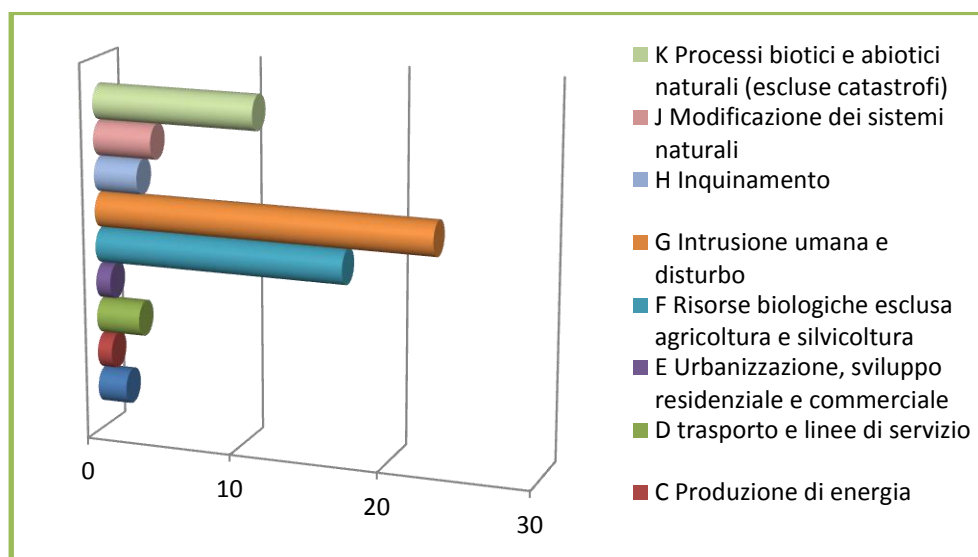
Figura 13. Pericoli e minacce nei siti controllati per le tre specie.
