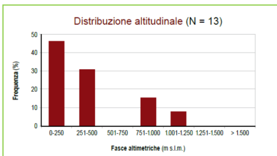
Figura 8. Distribuzione altitudinale del Lanario nel Lazio (Brunelli et al. , 2011).
