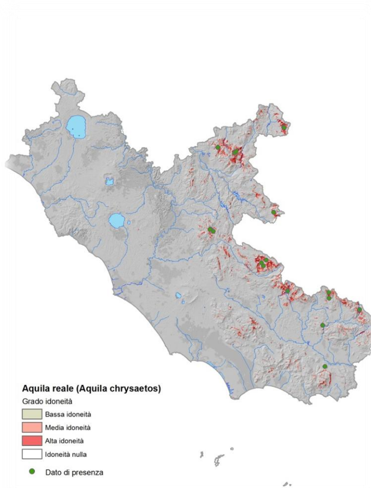
Figura 3. Modello di idoneità ambientale dell'Aquila reale nel Lazio realizzato attraverso il software MaxEnt (Sarrocco et al. , 2013).
