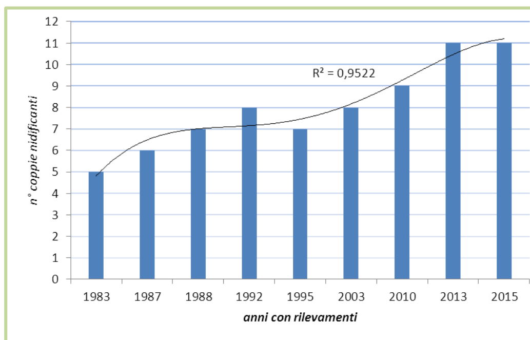
Figura 5. Evoluzione della popolazione nidificante di Aquila reale nel Lazio nel periodo 1983-2015. E' riportata la linea di tendenza e il valore del coefficiente R.
