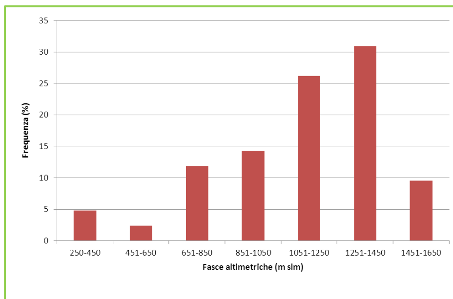
Figura 4. Distribuzione altitudinale dell'Aquila reale nel Lazio (Borlenghi et al. , 2014)).
