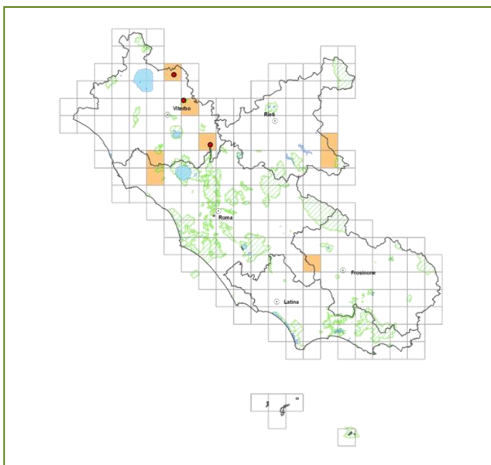
Figura 6. Distribuzione del Lanario nel Lazio nel periodo 2000-2009 (Aradis et al. , 2012)
