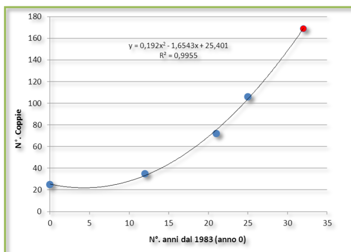
Figura 12. Evoluzione della popolazione di Falco pellegrino nel Lazio nel periodo 1983-2015. E' riportata la linea di tendenza, il coefficiente R e l'equazione della curva visualizzata. Il piccolo cerchio in rosso evidenzia il valore stimato con l'analisi di regressione.
