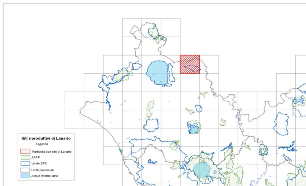
Figura 7. Localizzazione dell'unico sito riproduttivo di Lanario nel Lazio (aggiornamento 2015).
