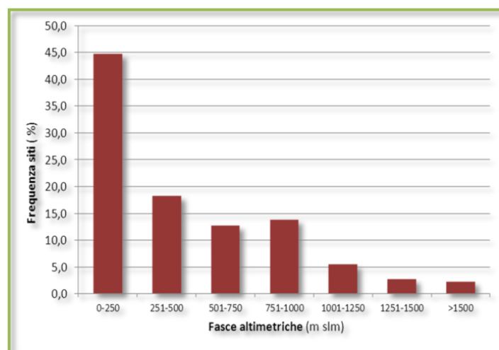
Figura 11. Distribuzione altitudinale del Falco pellegrino nel Lazio, siti 2008-2015.
