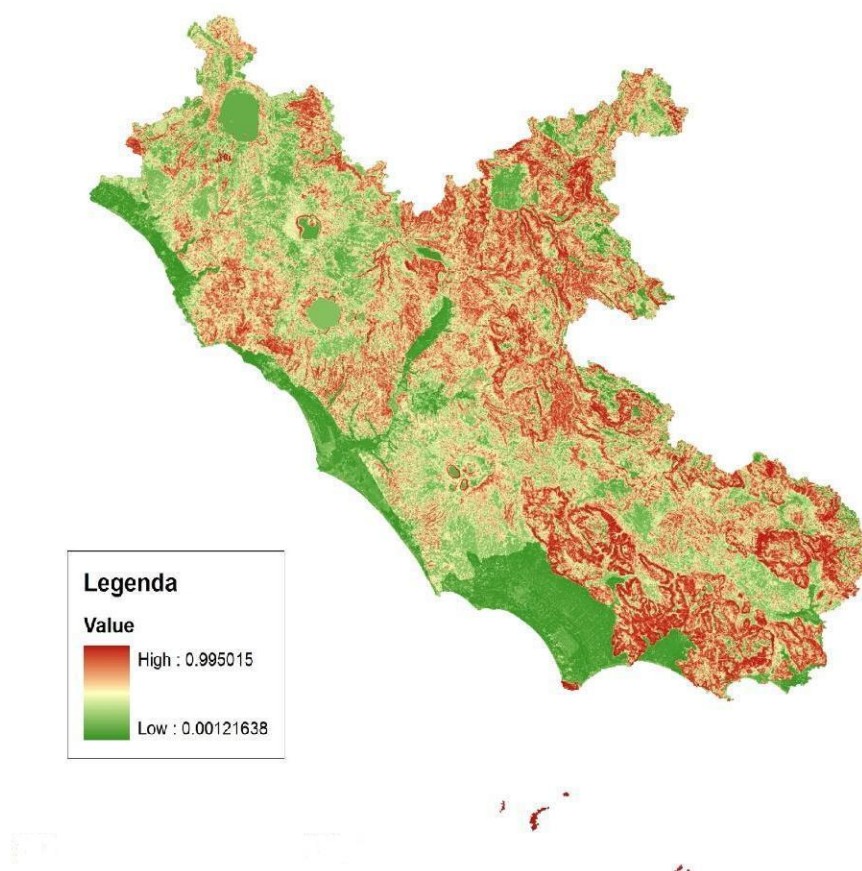
Figura 12. Modello di idoneità ambientale del Pellegrino nel Lazio (Pezzarossa, 2014-15)
